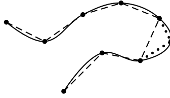
Slika 1. Aproximacija gladke krivulje s poligonalno.
